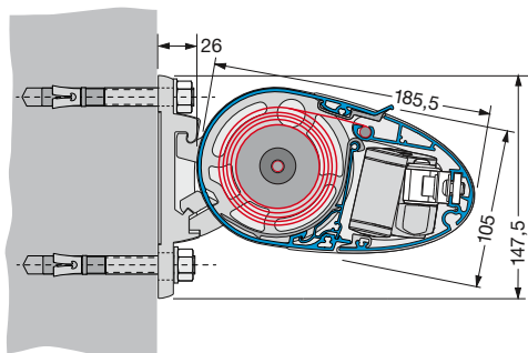
Ściana
