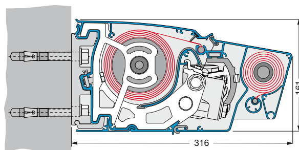
Ściana
