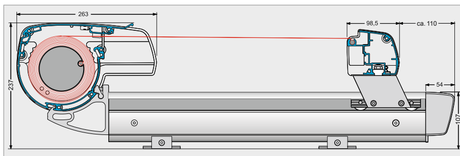
Stopka montażowa (różne wysokości)
