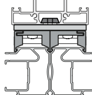
Stopka montażowa z podwójnym uchwytem, z płytki dociskową do montażu na szklanym dachu Murano
