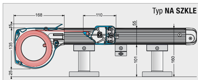
Stopka montażowa z podwójnym uchwytem, z płytki dociskową do montażu na szklanym dachu Murano
