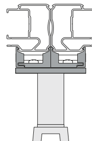
Stopka montażowa z podwójnym uchwytem
