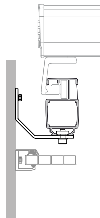
Mocowanie boczne do ściany
