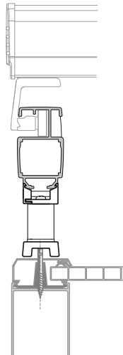
Stopka montażowa (różne wysokości)
